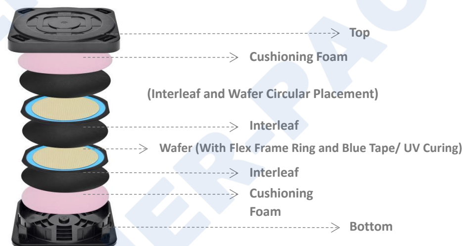
* FHWS-8/13
