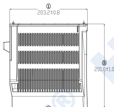
* MCS-8/25-NP-PFA
