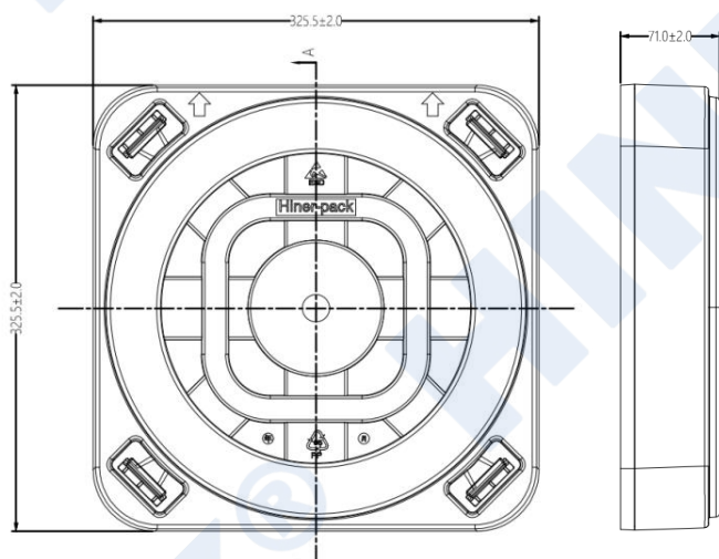
* FHWS-8/13
