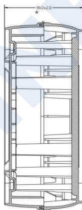
SECTION A-A
